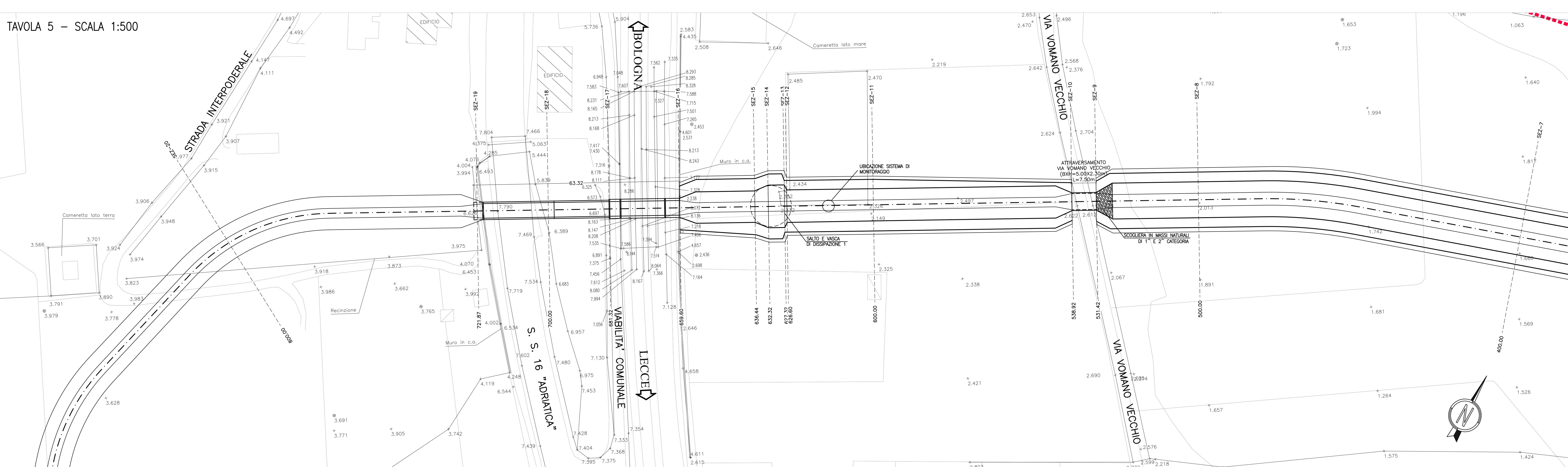
TAVOLA 6 - SCALA 1:500
